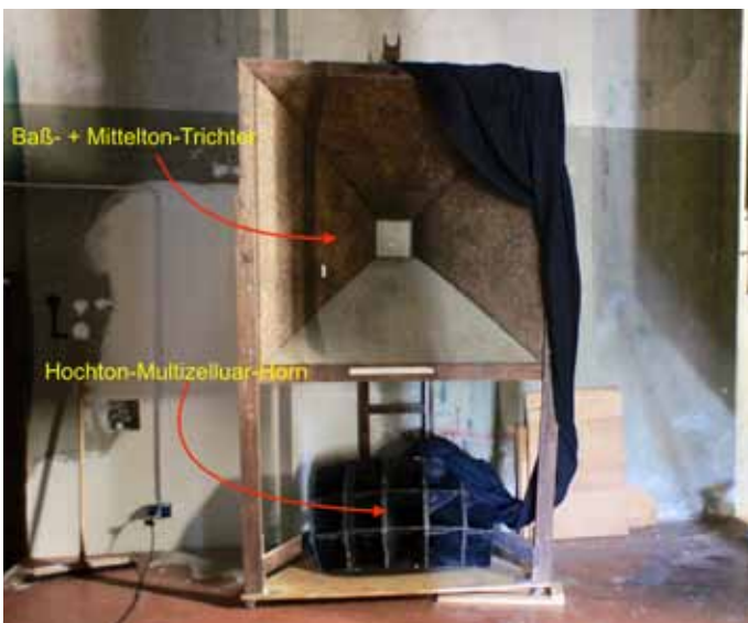
Fundzustand des Bühnenlautsprechers.
